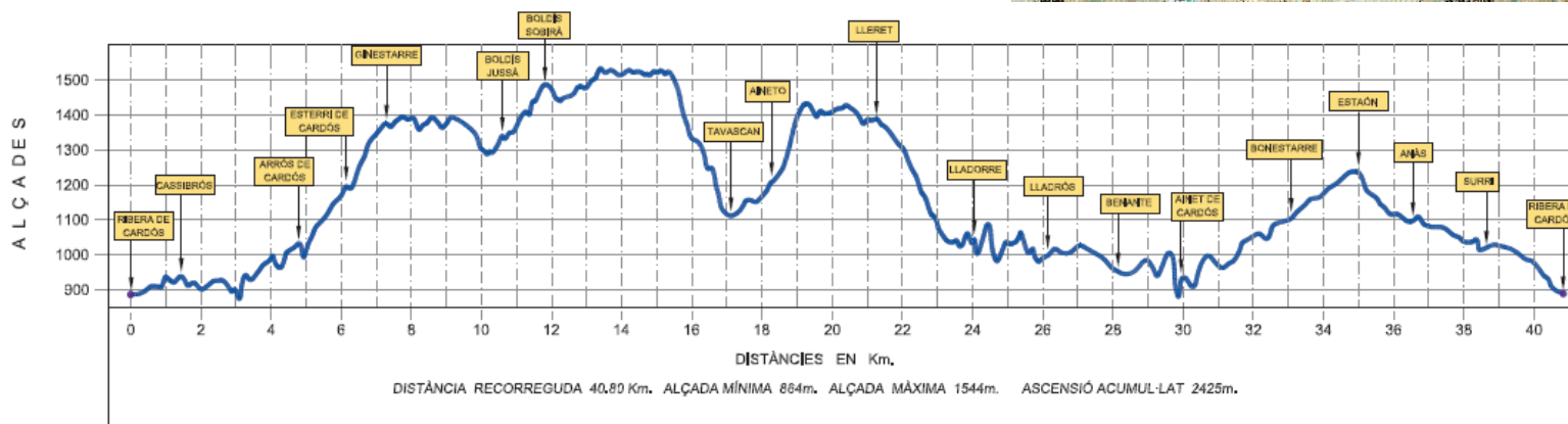
PERFIL LONGITUDINAL PER DISTÀNCIES
